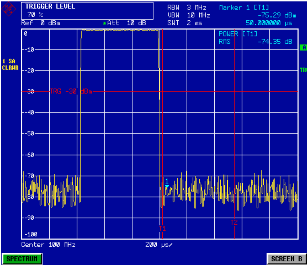
Bild 5-15 Messung des Signal-/Rauschverhältnisses eines GSM-Burst-Signals im Zeitbereich
