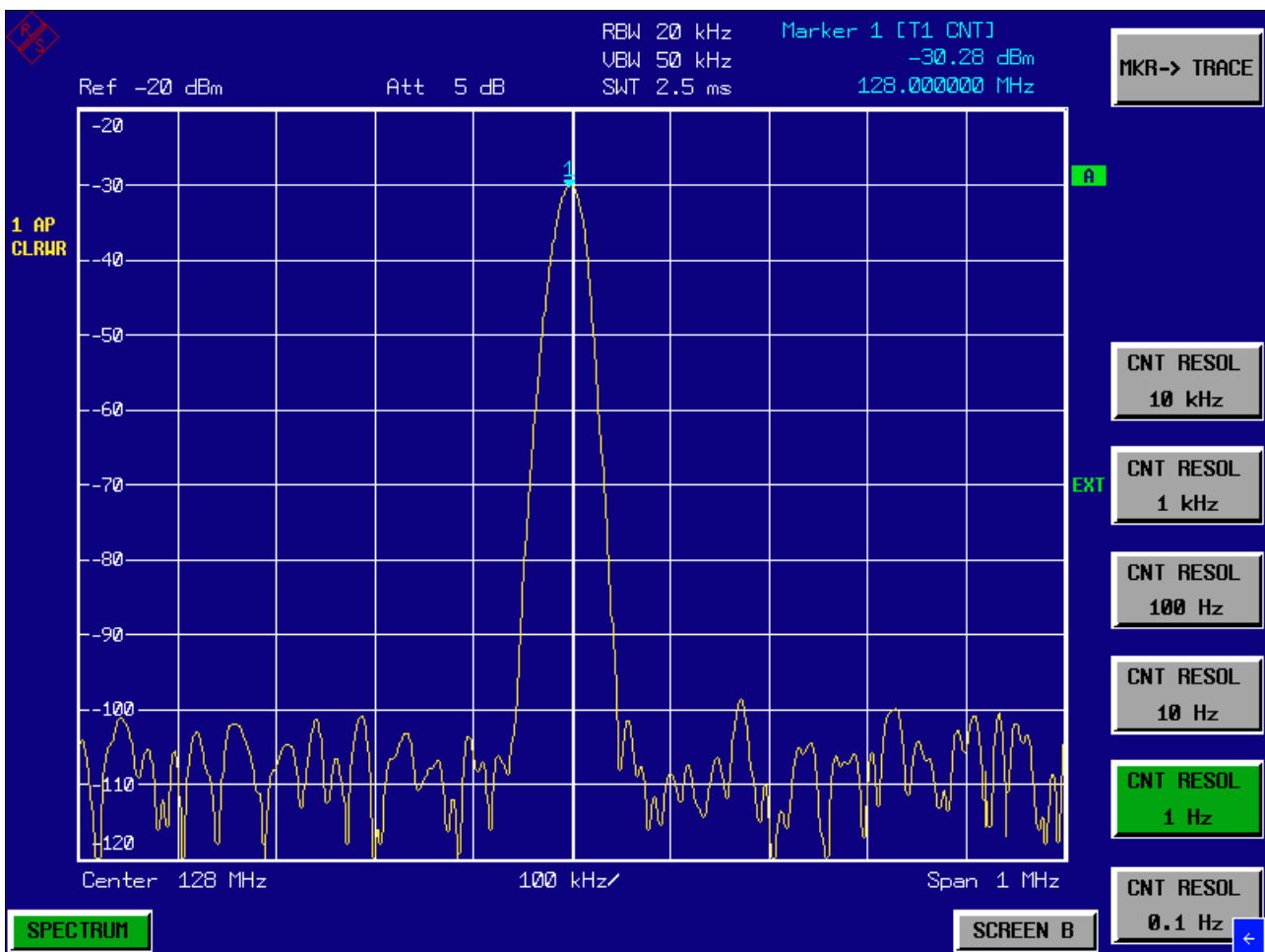
Bild 5-1 Messung der Frequenz mit dem Frequenzzähler
