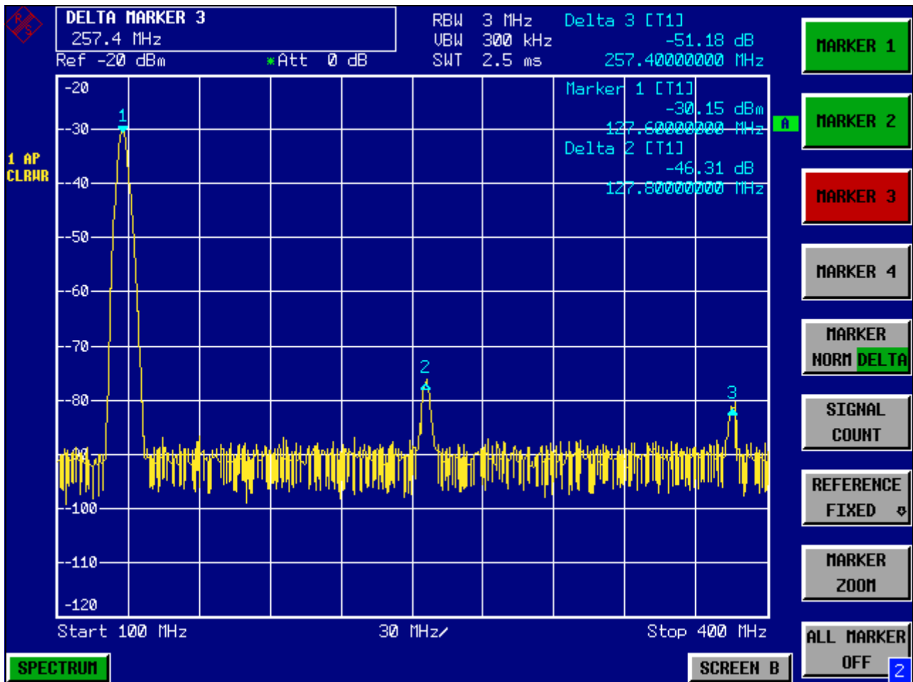
Bild 5-2 Messung des Harmonischenabstands des internen Referenzgenerators. Die Marker Delta 2 [T1] und Delta 3 [T1] zeigen den Abstand der ersten und zweiten Oberwelle zur Grundwelle an.
