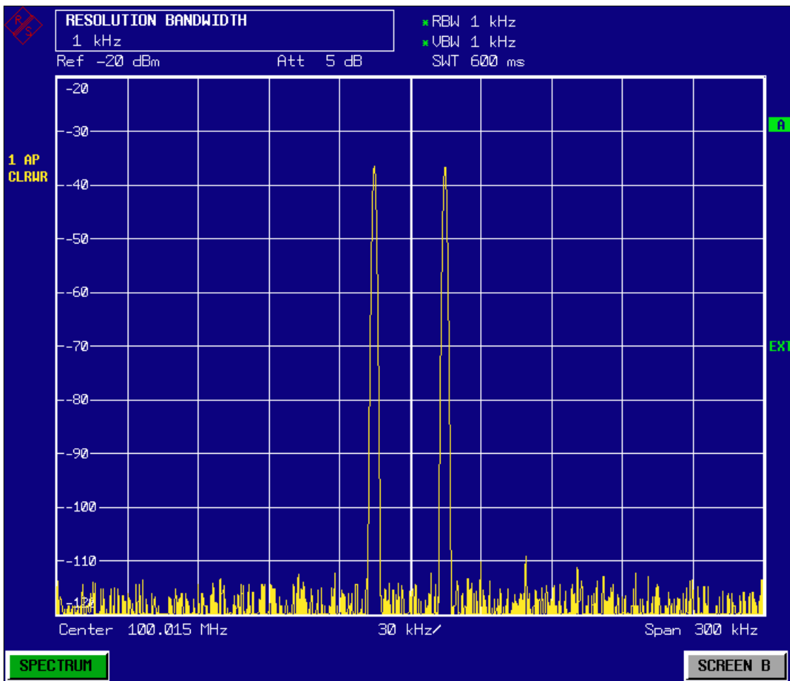
Bild 5-8 Messung von zwei gleich großen HF-Sinussignalen mit einer Auflösebandbreite (1 kHz), die deutlich kleiner ist als deren Frequenzabstand.
