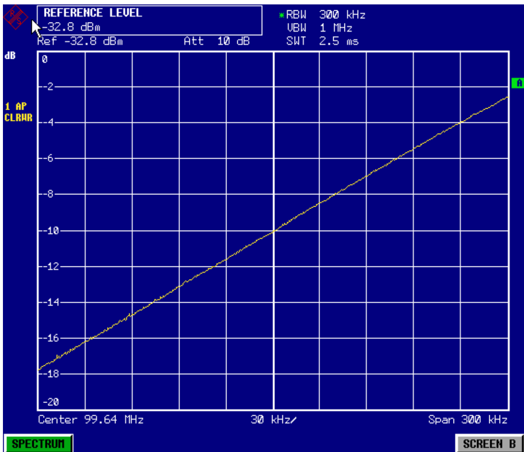
Bild 5-17 Darstellung der Filterflanke des 300-kHz-Filters als FM-Diskriminatorekennlinie.
