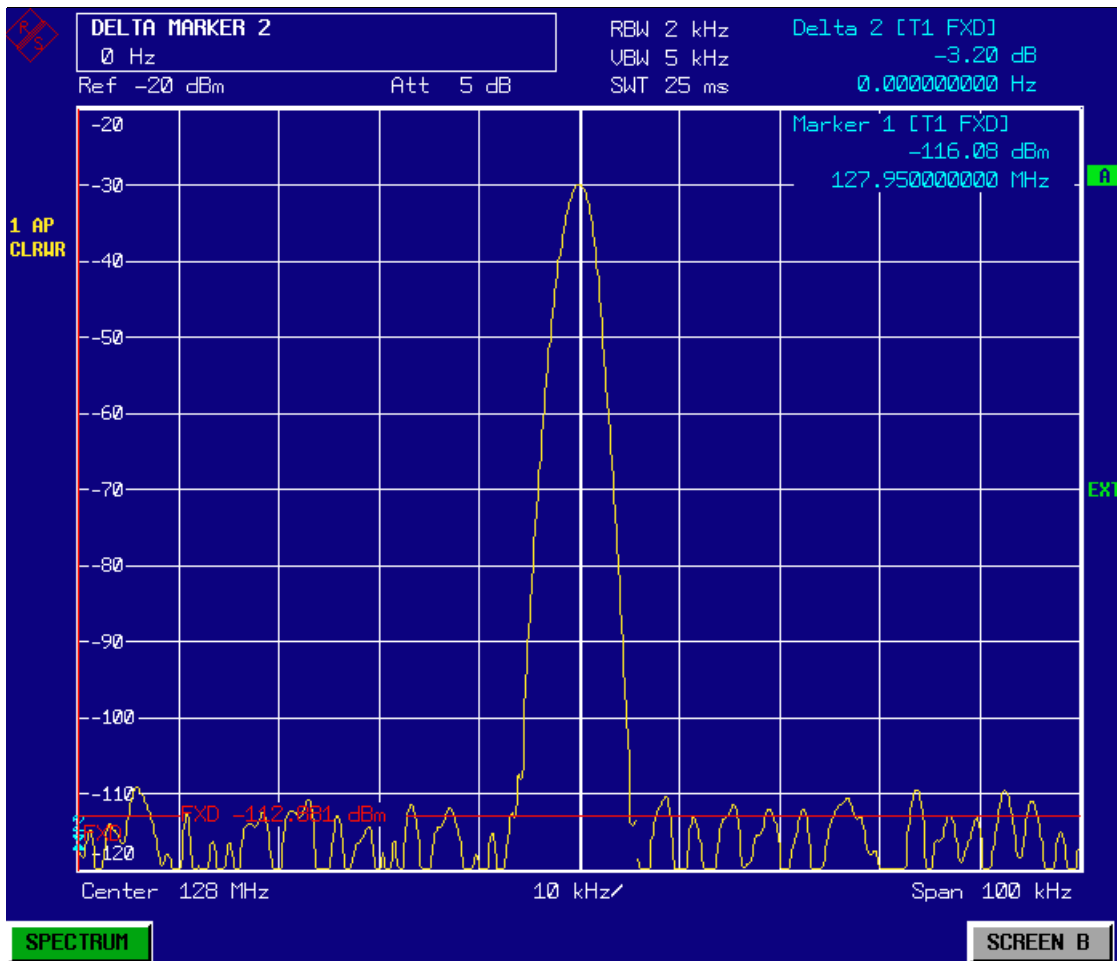
Bild 5-4 Darstellung der Grundwelle mit dem Bezugspunkt für Frequenz und Pegel
