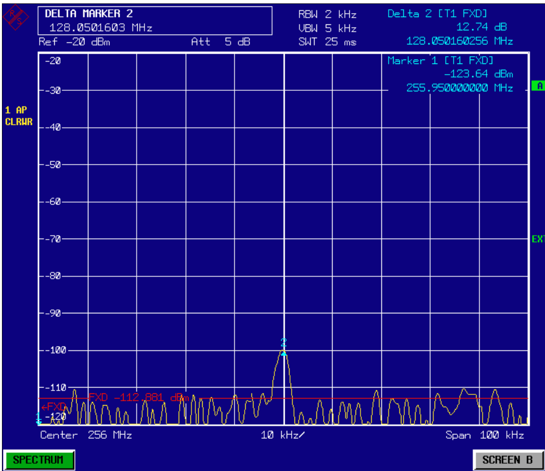
Bild 5-5 Messung des Pegelabstands der 1. Oberwelle (Abstand zum Bezugspegel = Pegel des 1. Harmonische)
