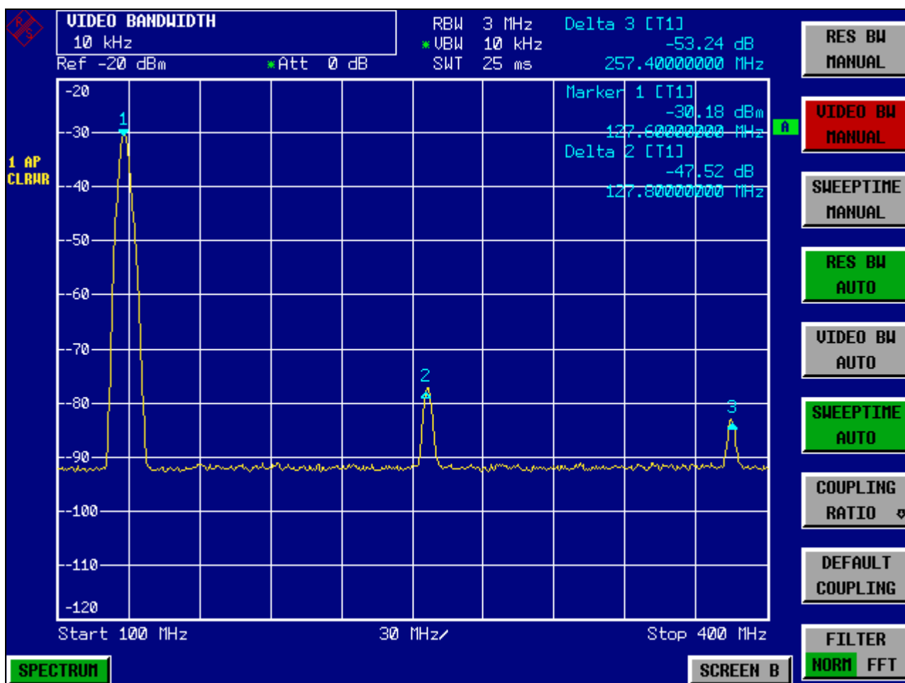
Bild 5-3 Unterdrückung des Rauschens bei der Oberwellenmessung durch Verringerung der Videobandbreite
