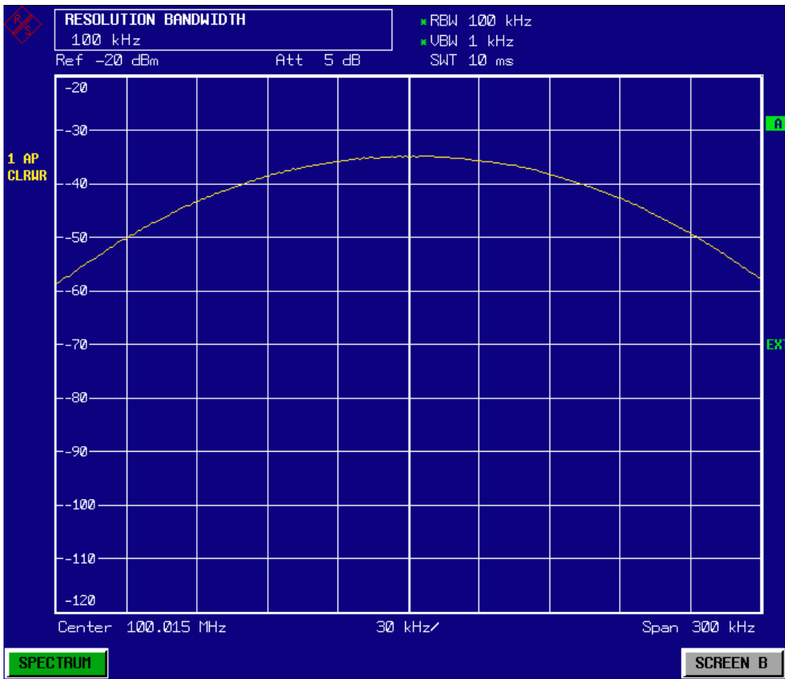
Bild 5-7 Messung von zwei gleich großen HF-Sinussignalen mit einer Auflösebandbreite, die größer als deren Frequenzabstand ist.
