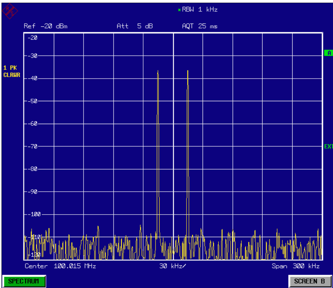
Bild 5-9 Messung mit FFT-Filtern ergibt eine erheblich kürzere Sweep-Zeit und eine höhere Aktualisierungsrate.
