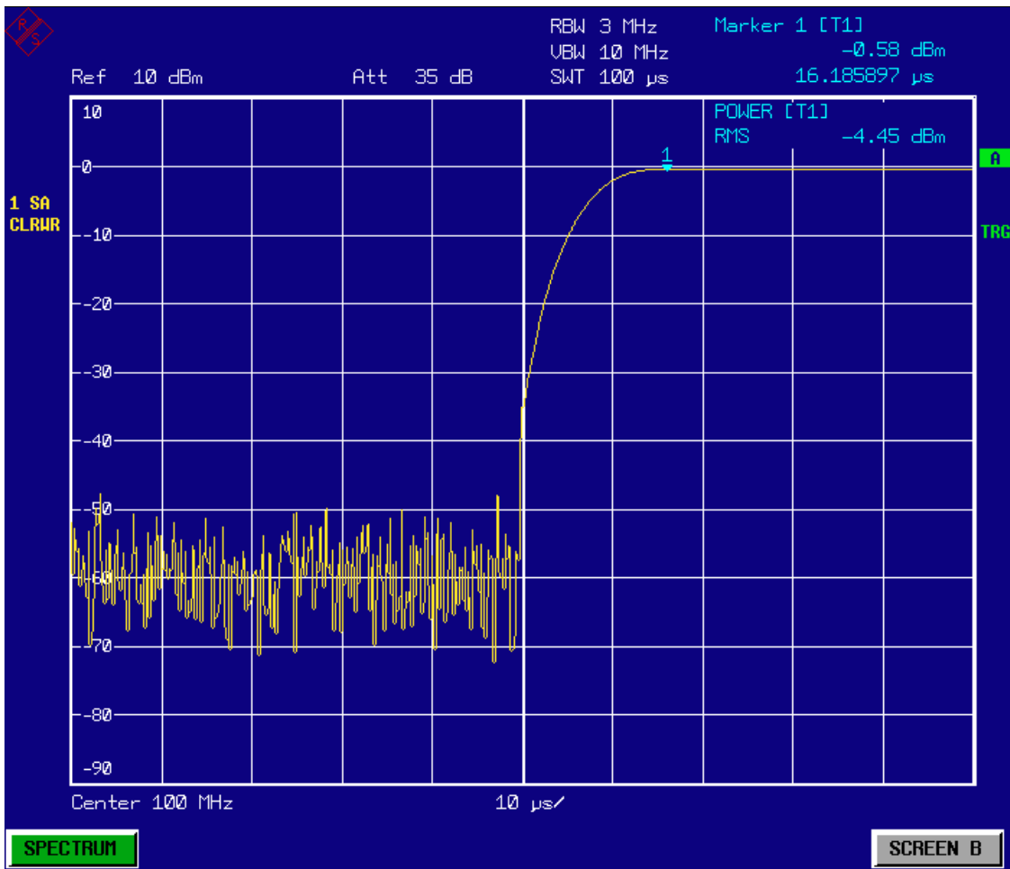
Bild 5-12 Steigende Flanke des GSM-Bursts mit hoher Zeitauflösung dargestellt.
