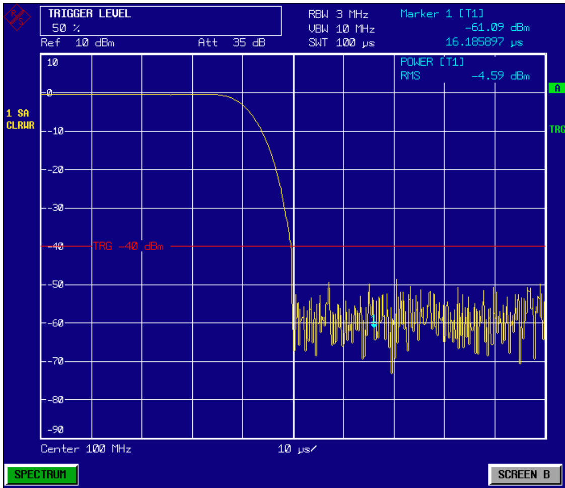
Bild 5-13 Fallende Flanke des GSM-Bursts mit hoher Zeitaufösung dargestellt.
