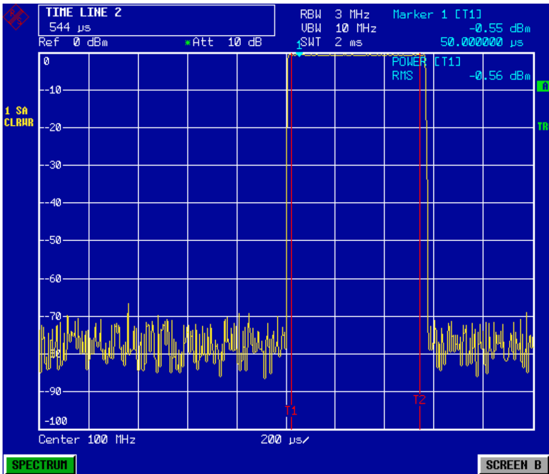
Bild 5-14 Messung der Leistung während der Einschaltphase des Bursts
