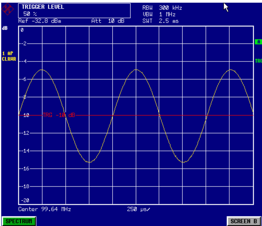
Bild 5-18 Darstellung des demodulierten FM-Signals
