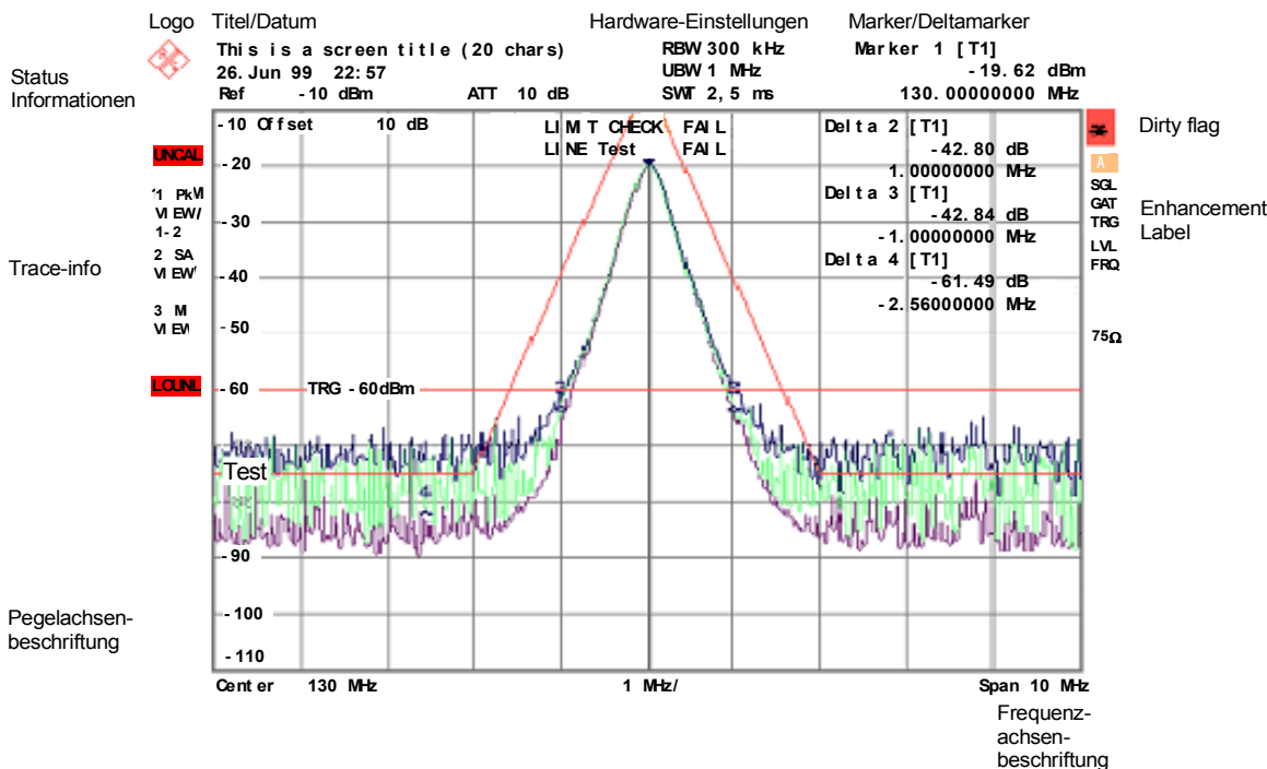
Bild 4-1 Bildschirmaufteilung des R&S FSU im Analysatorbetrieb
