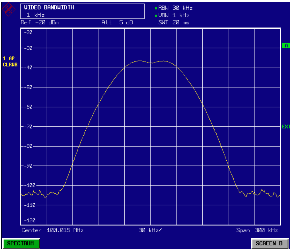
Bild 5-6 Messung von zwei gleich großen HF-Sinussignalen mit einer Auflösebandbreite, die dem Frequenzabstand der Signale entspricht.
