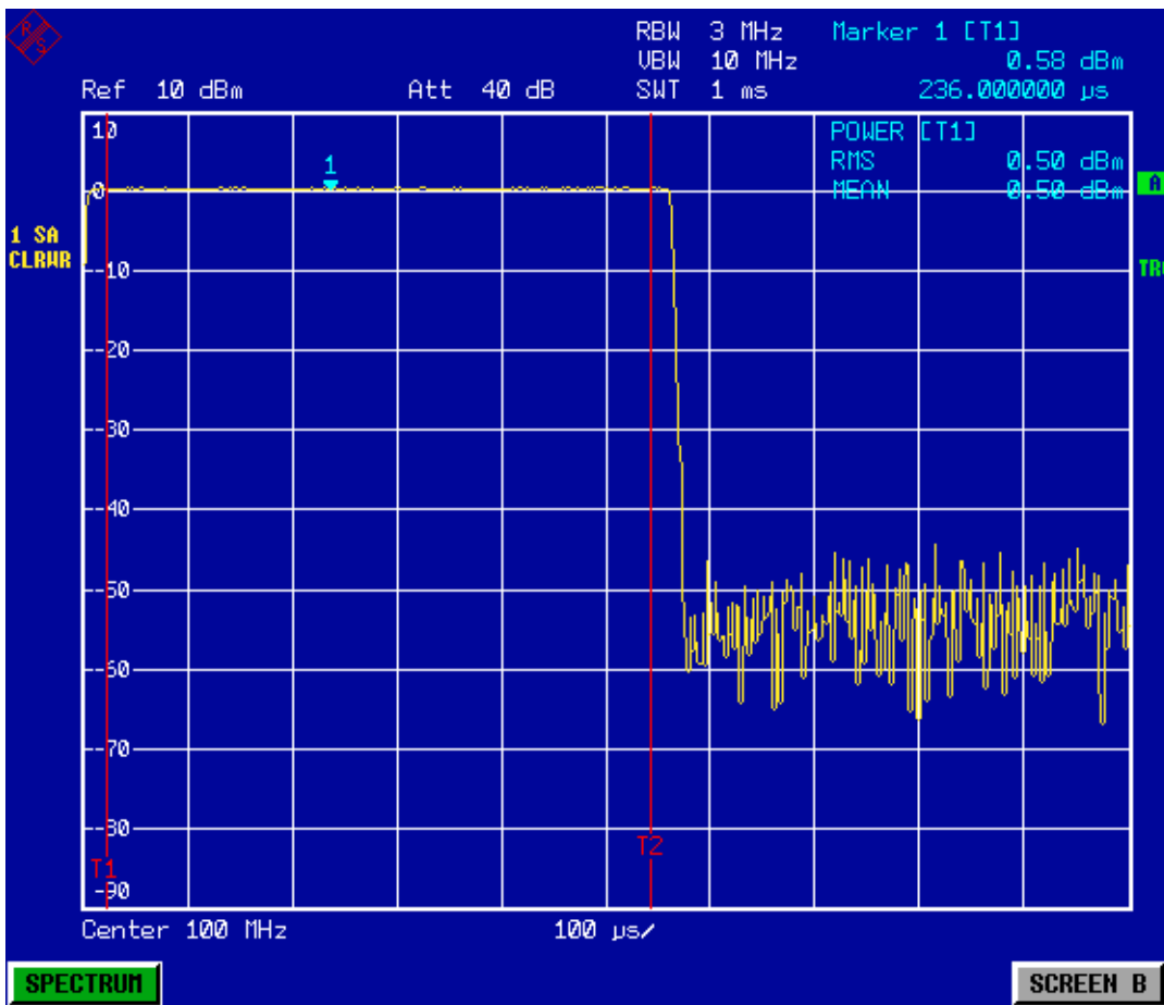
Bild 5-11 Messung der mittleren Leistung eines GSM-Bursts.
