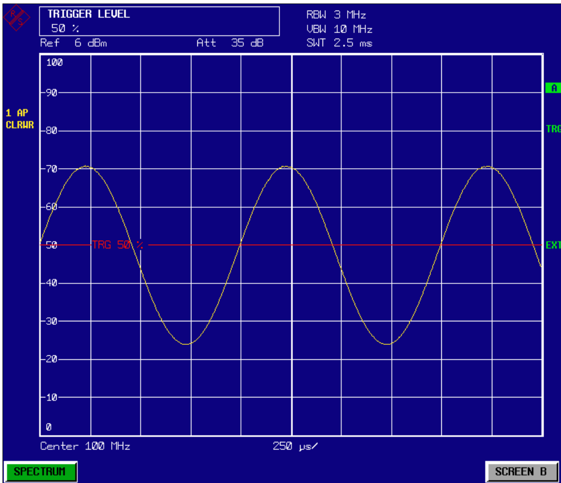
Bild 5-16 Messung des NF-Signals eines mit 1 kHz AM-modulierten Trägers Die NF mit dem eingebauten Lautsprecher abgehört werden.
